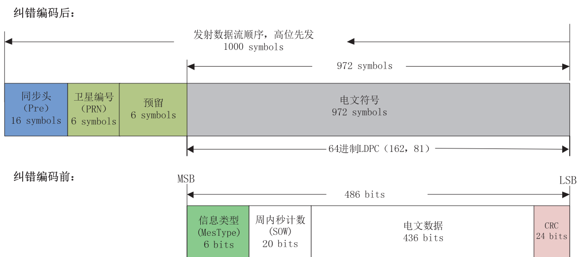
图 6-1 B-CNAV3 帧结构
