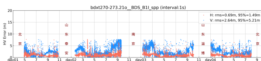
图 7 北斗系统 B1I 定位误差时间序列
