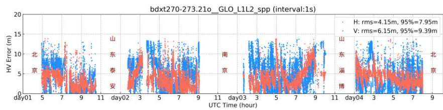
图 16 GLONASS L1L2 双频定位误差时间序列
