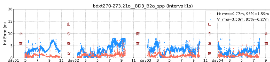
图 11 北斗系统 B2a 定位误差时间序列
