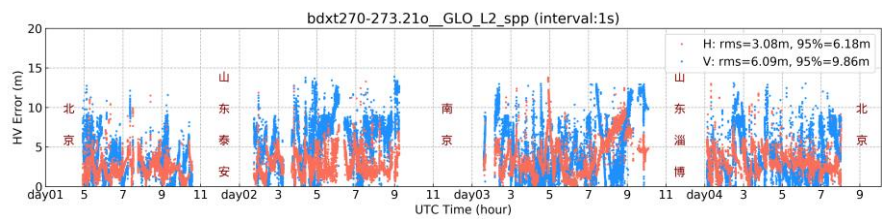
图 15 GLONASS L2 定位误差时间序列
