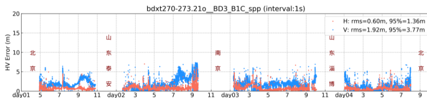
图 10 北斗系统 B1C 定位误差时间序列
