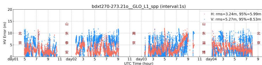
图 14 GLONASS L1 定位误差时间序列
