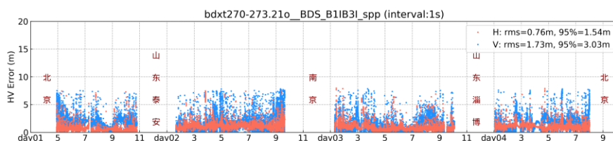
图 9 北斗系统 B1I&B3I 双频定位误差时间序列
