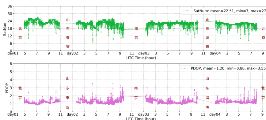
图 5 测试中北斗 B1I/B3I/B1IB3I 频点可见卫星数和 PDOP
