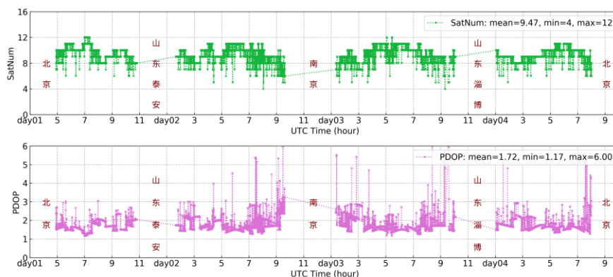
图 6 测试中北斗 B1C/B2a/B1CB2a 频点可见卫星数和 PDOP
