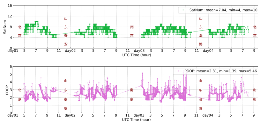
图 13 测试中 GLONASS 可见卫星数目及 DPOP 值
