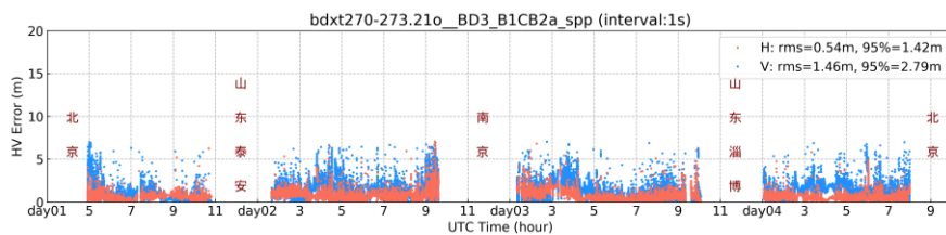
图 12 北斗系统 B1CB2a 双频定位误差时间序
