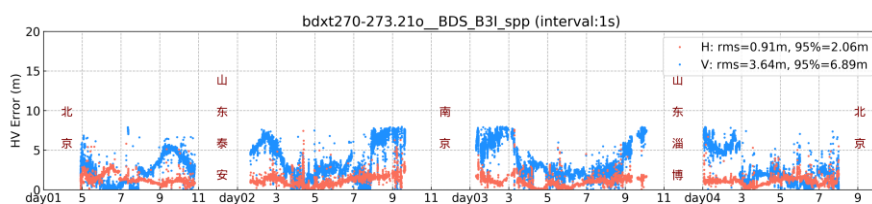
图 8 北斗系统 B3I 定位误差时间序列
