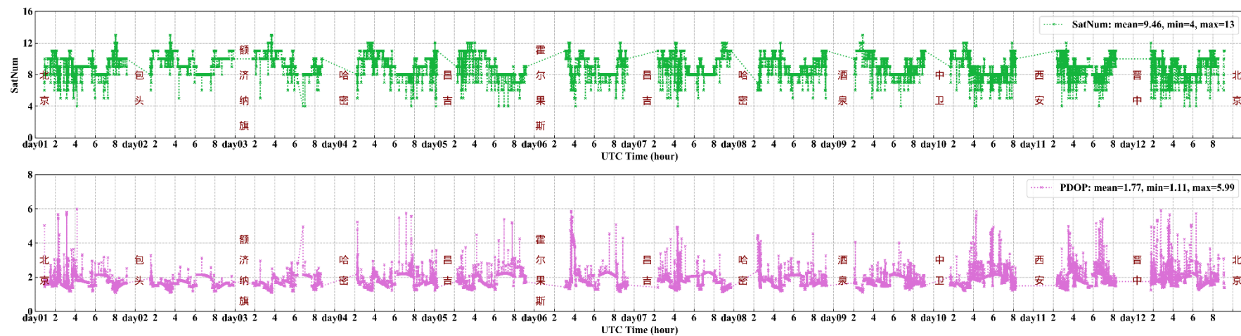
图 6 测试中北斗 B1C/B2a/B1C B2a 频点可见卫星数和 PDOP
