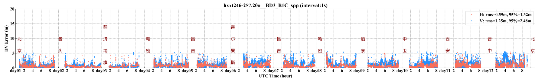
图 10 北斗系统 B1C 定位误差时间序列
