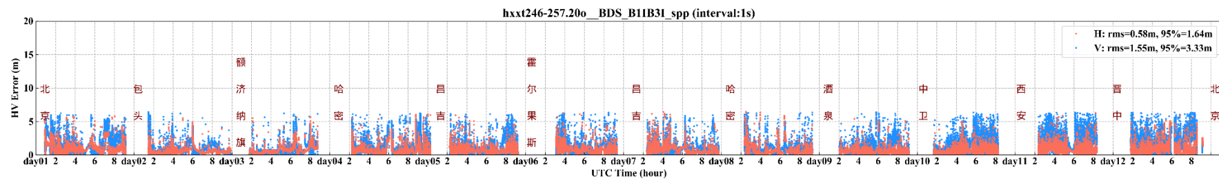
图 9 北斗系统 B1I&B3I 双频定位误差时间序列
