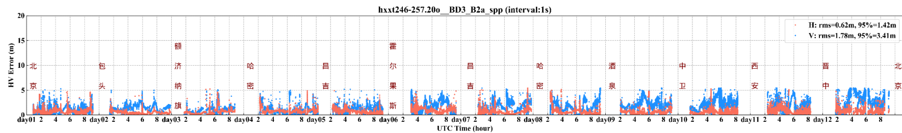
图 11 北斗系统 B2a 定位误差时间序列
