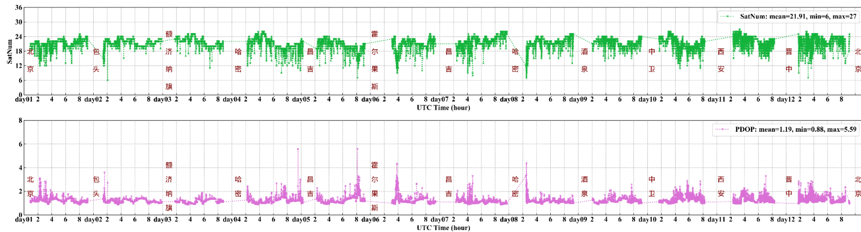
图 5 测试中北斗 B1I/B3I/B1I B3I 频点可见卫星数和 PDOP
