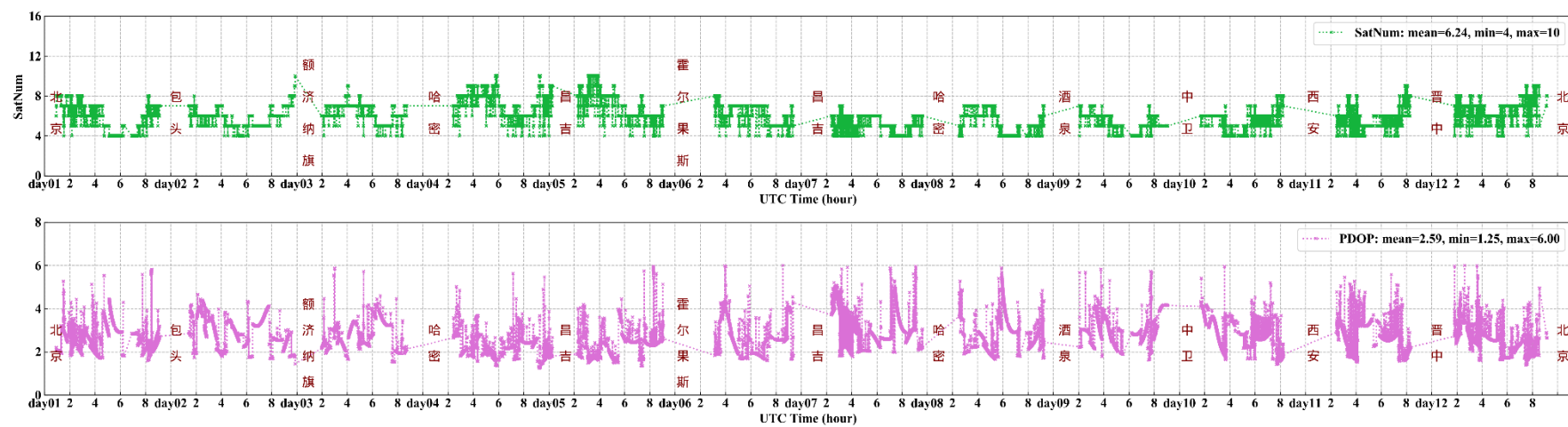
图 13 测试中 GLONASS 可见卫星数目及 DPOP 值
