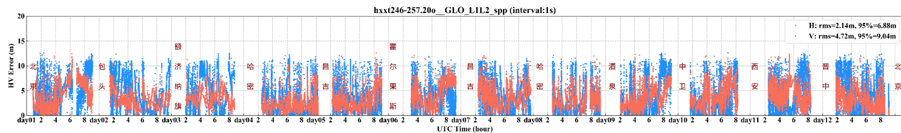
图 16 GLONASS L1L2 双频定位误差时间序列
