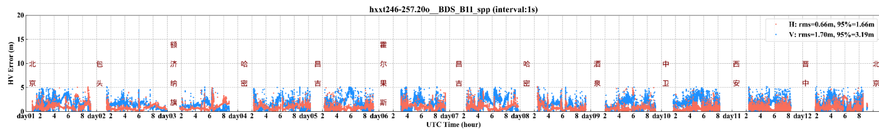
图 7 北斗系统 B1I 定位误差时间序列
