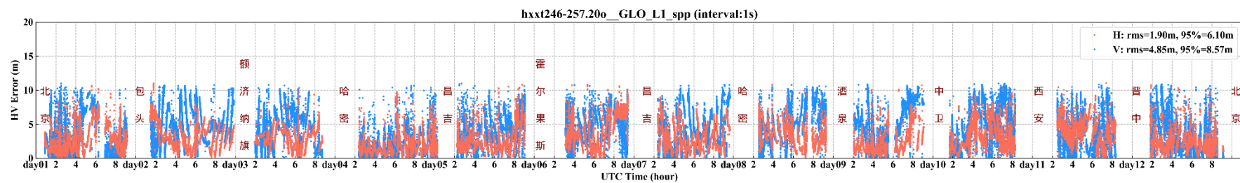
图 14 GLONASS L1 定位误差时间序列
